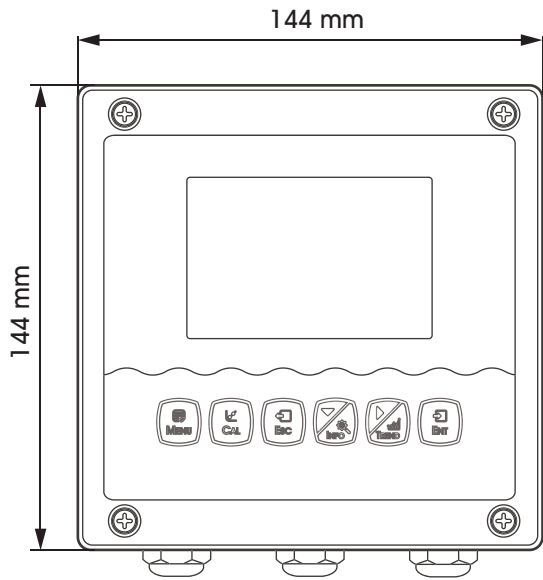
仪器外形尺寸
