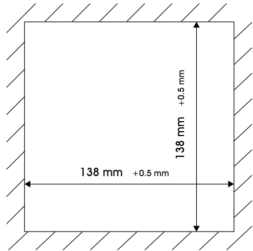
嵌入式安装开孔尺寸
